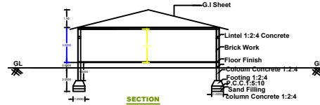
SECTION - AB
