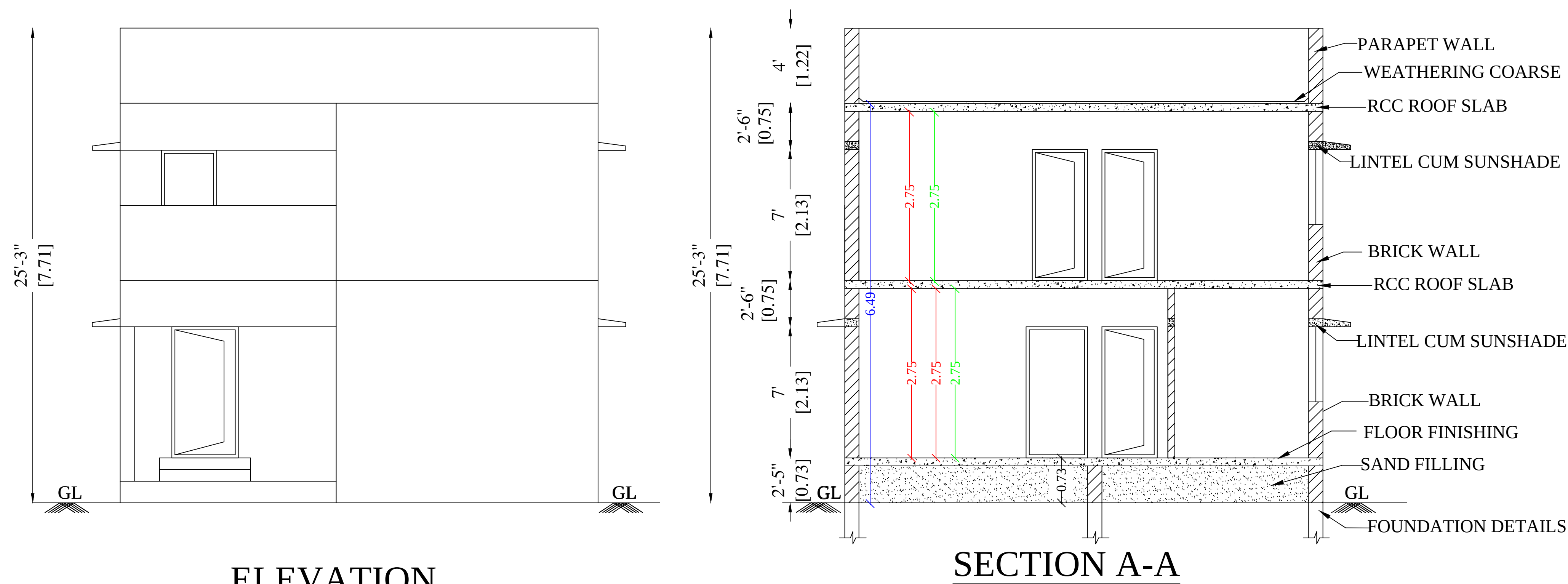
ELEVATION
