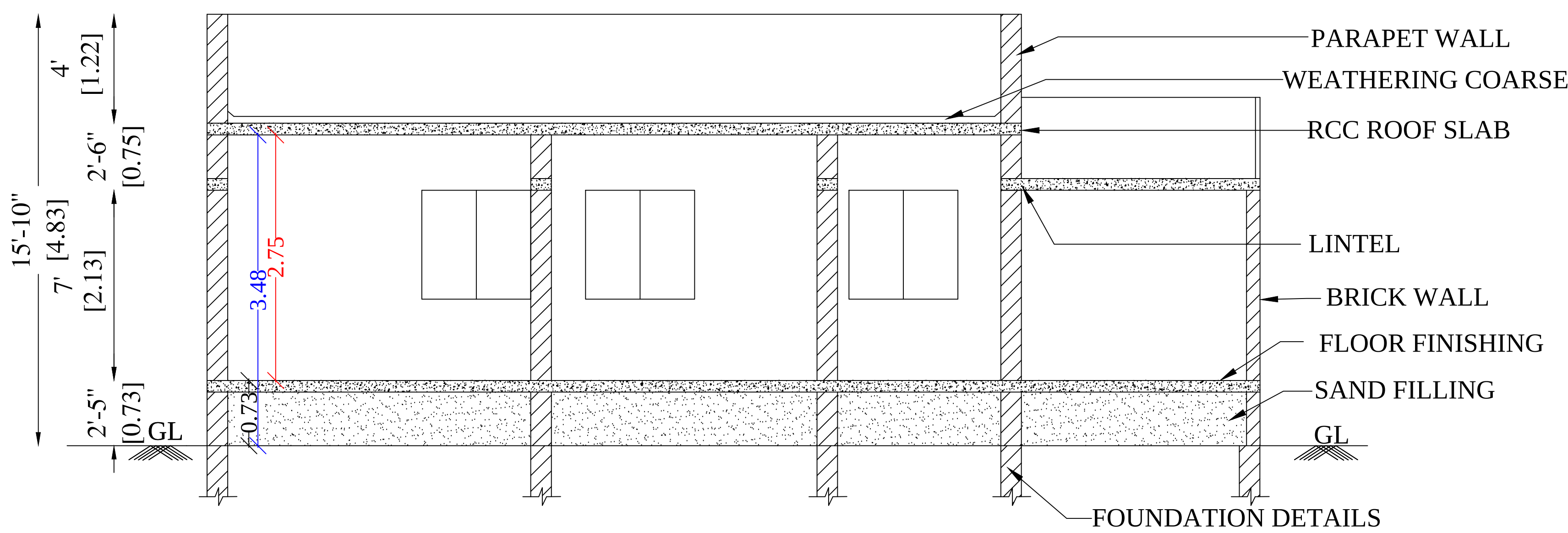
SECTION A-A
