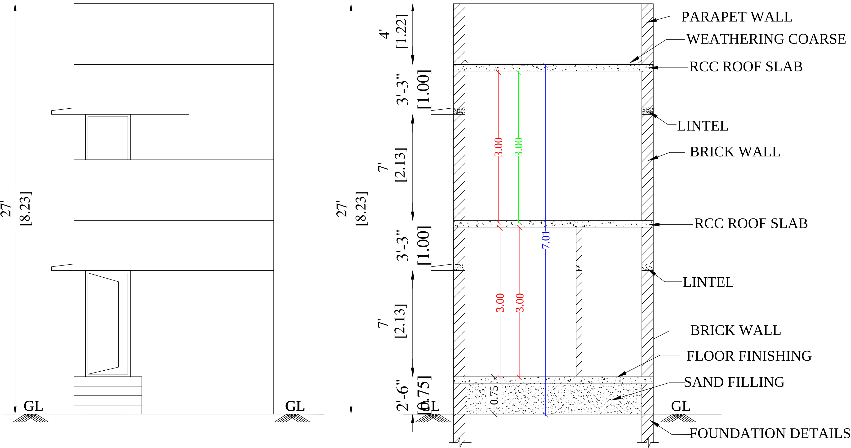
ELEVATION
