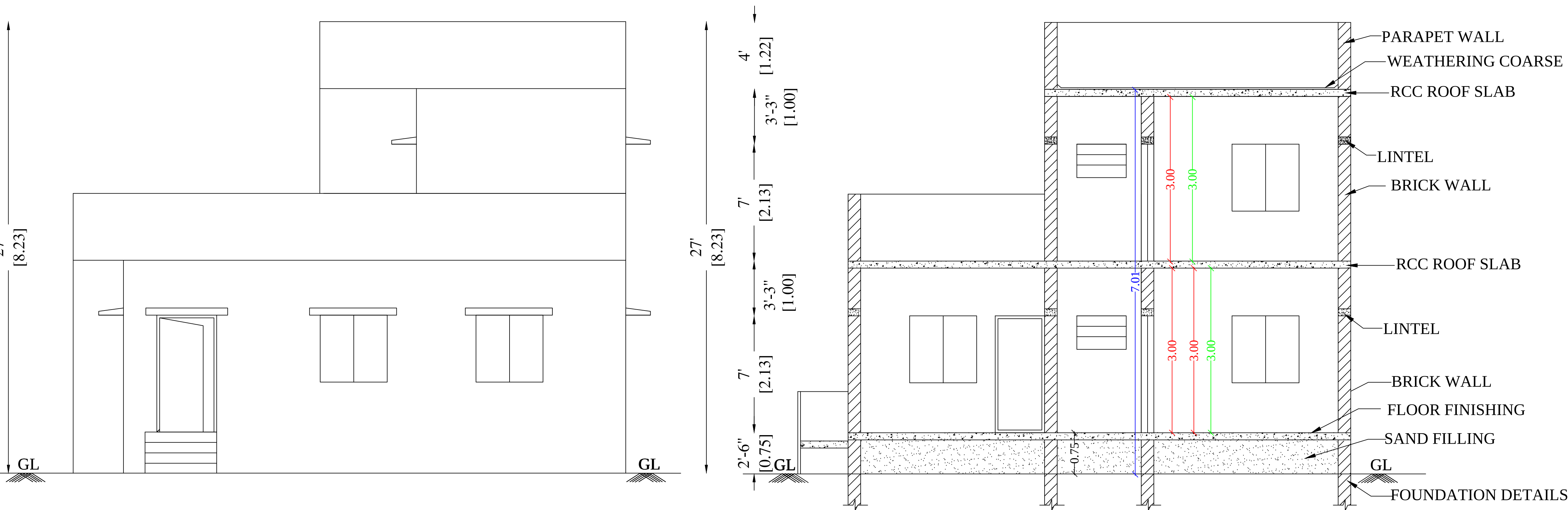
ELEVATION
