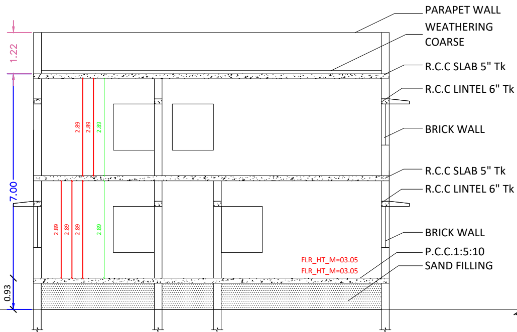
SECTION -AB
