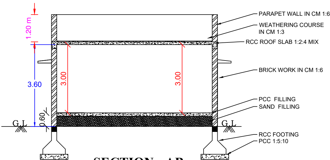
SECTION - AB
