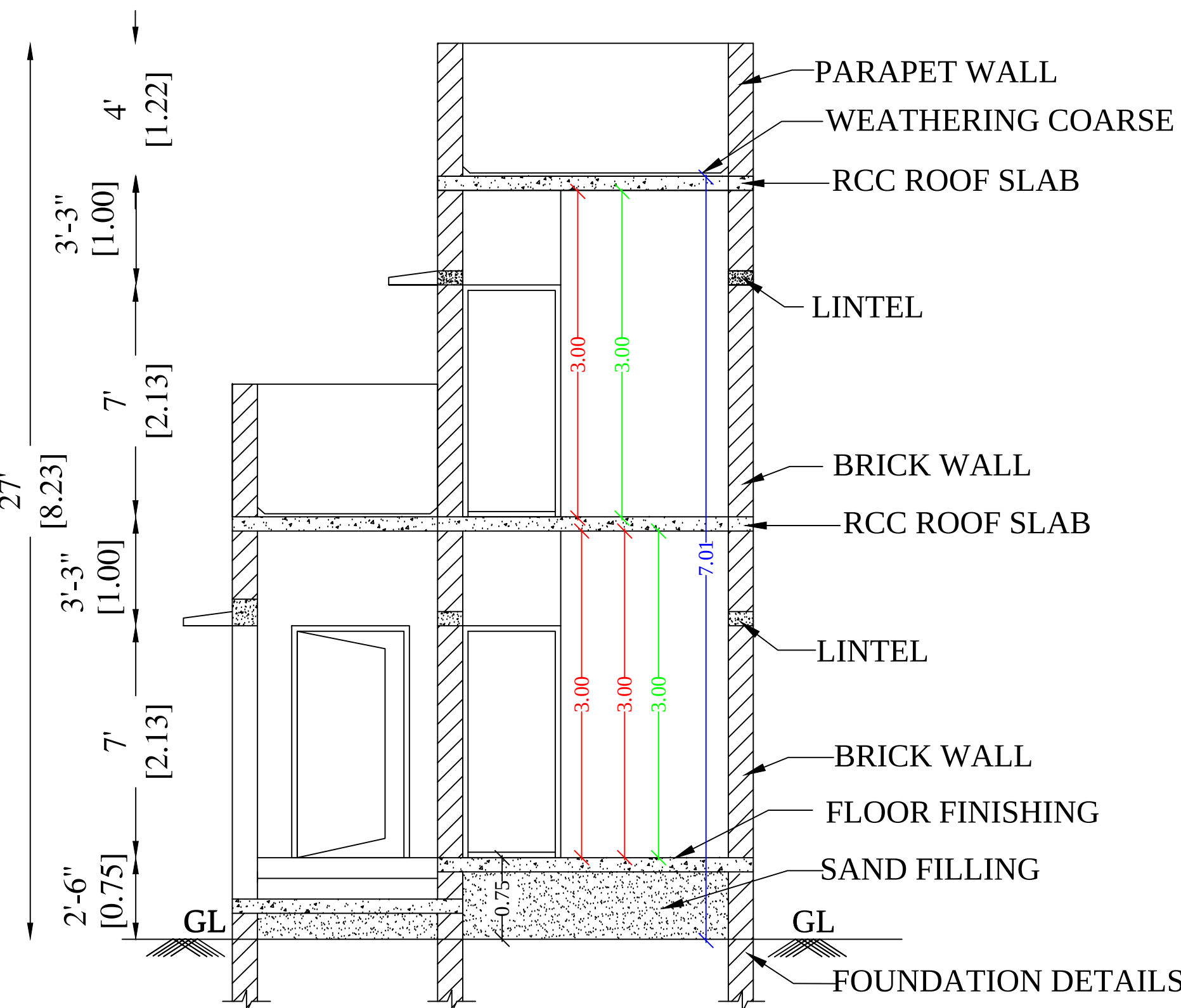
SECTION A-A
