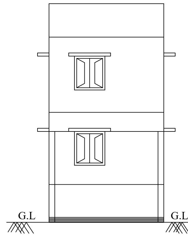
ELEVATION
