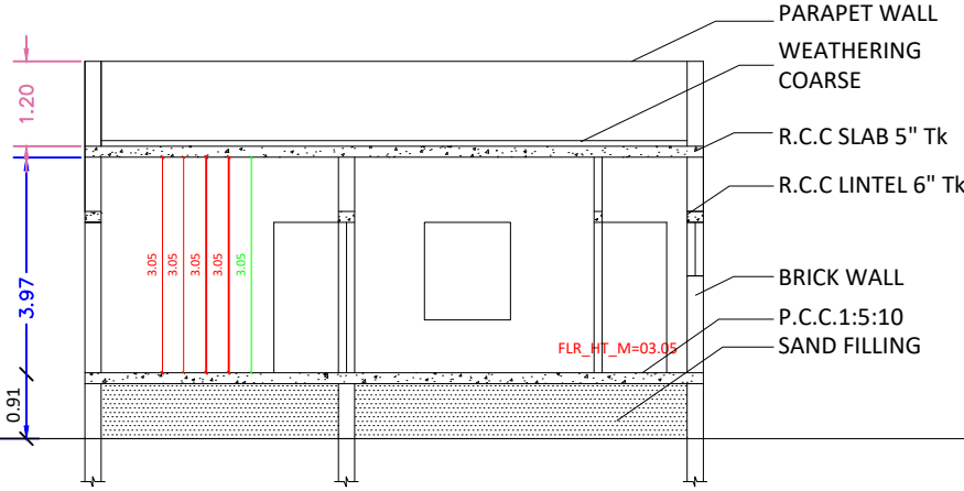
SECTION -AB
