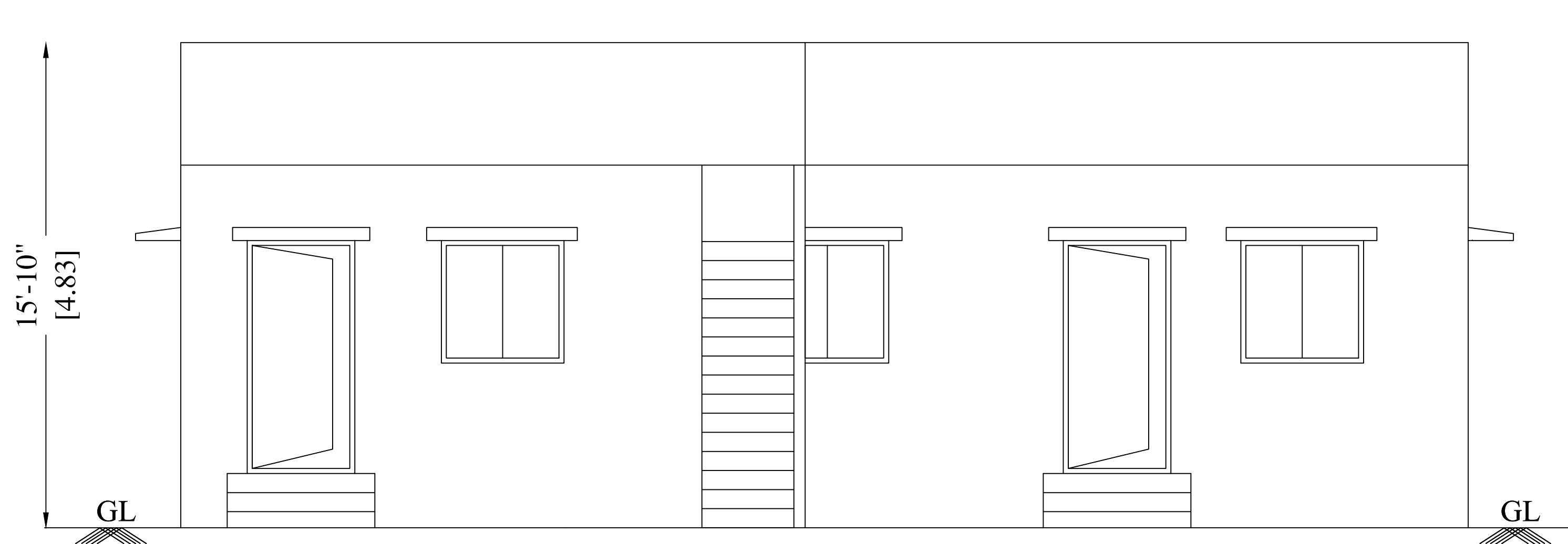
ELEVATION
