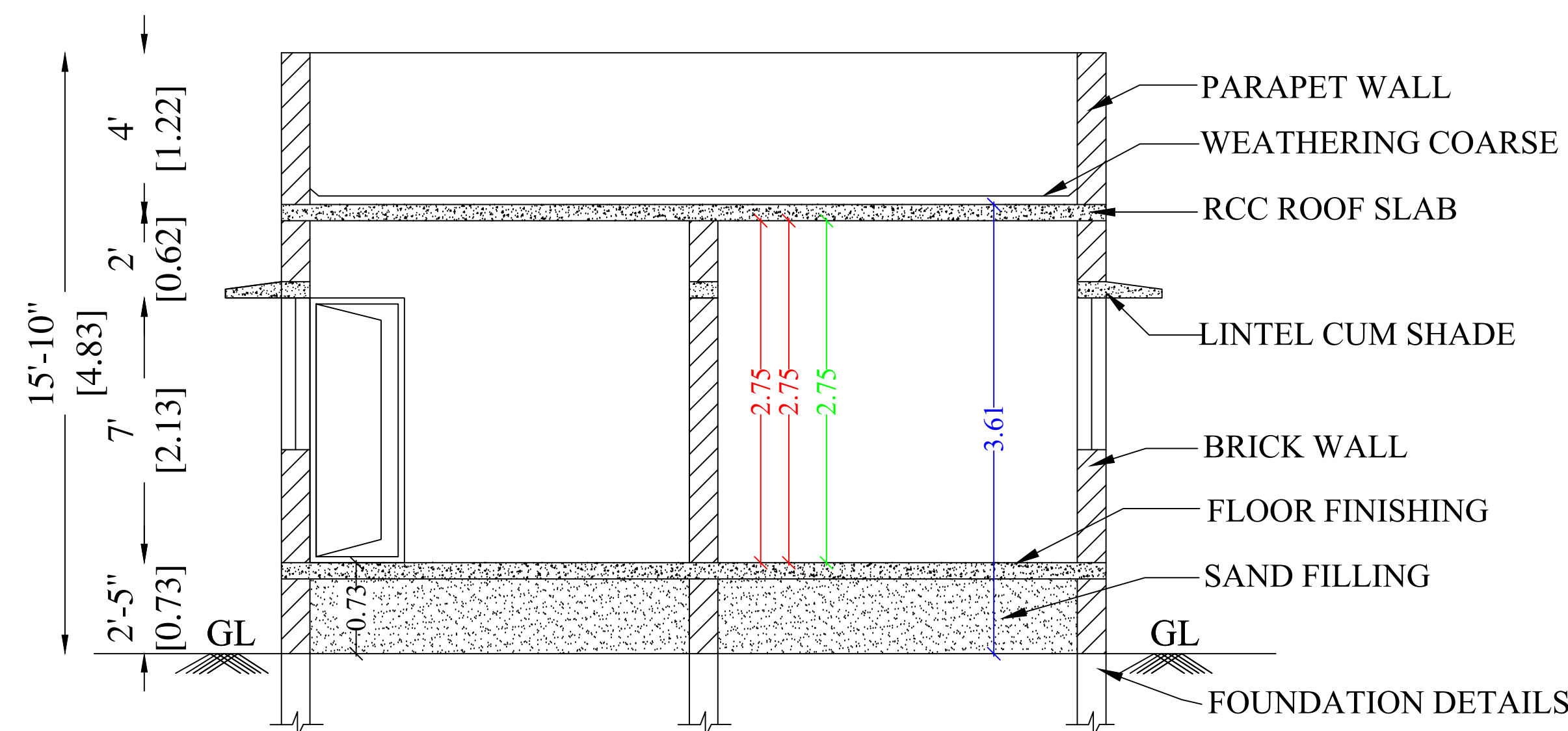
SECTION A-A
