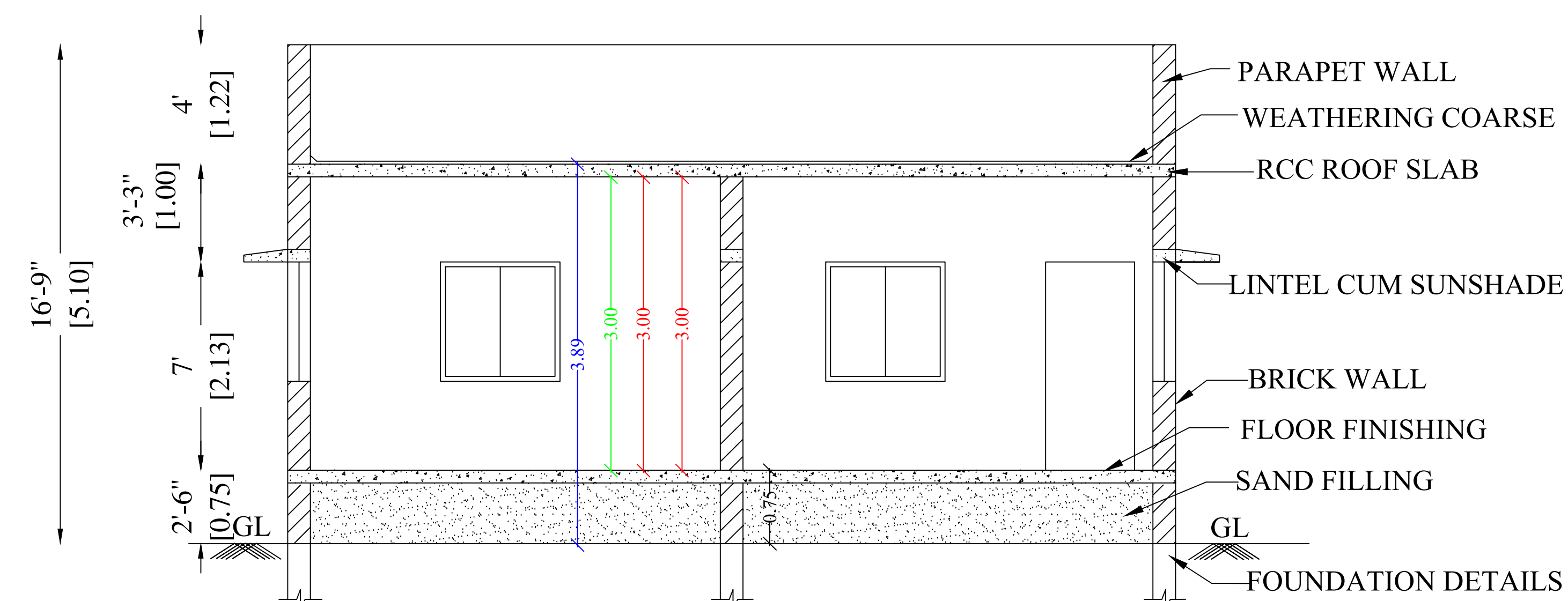
SECTION A-A
