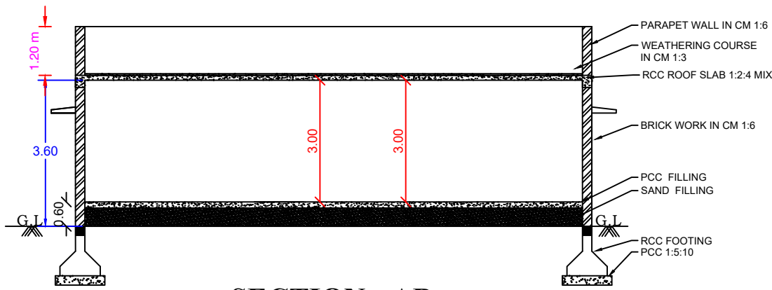
SECTION - AB
