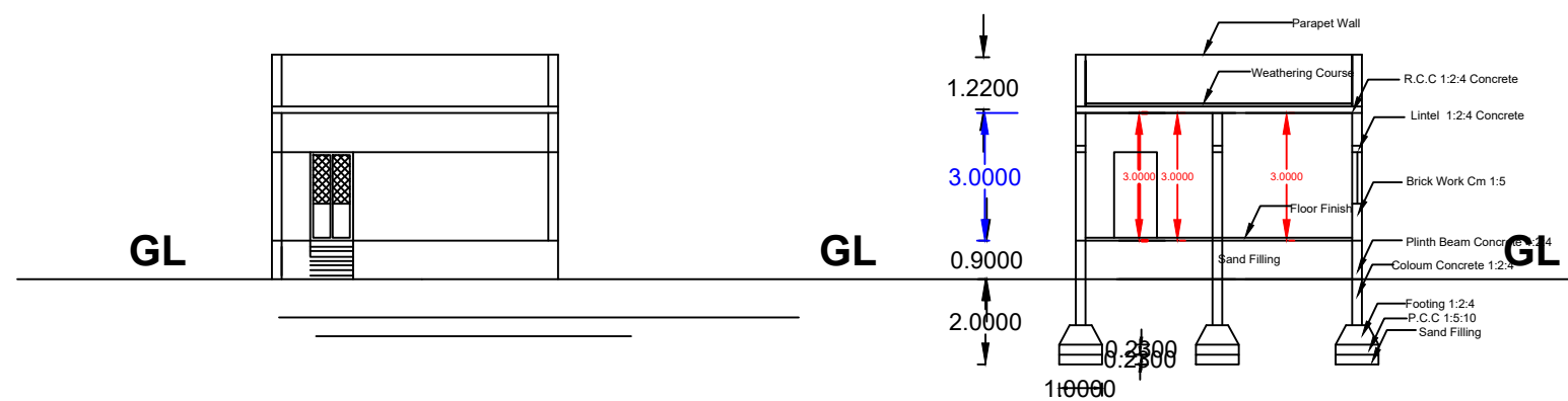
Elevation
