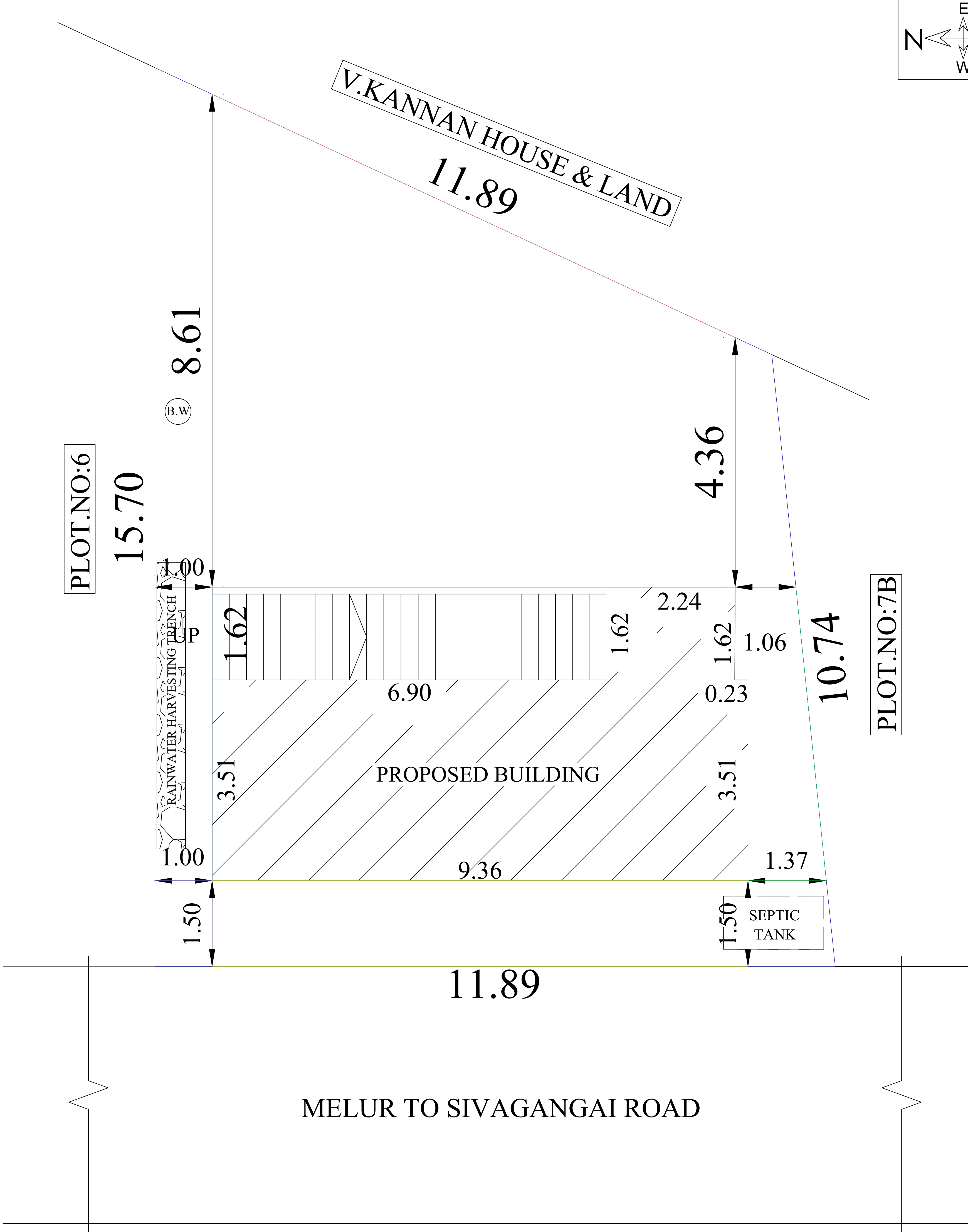
SITE PLAN 1:100
