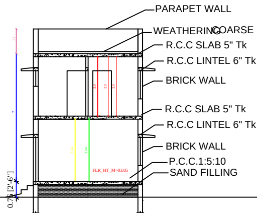
SECTION -AB
