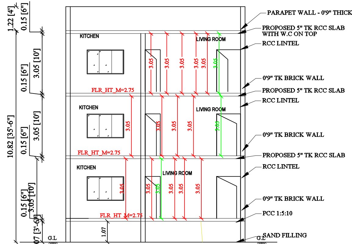
SECTION A-A
