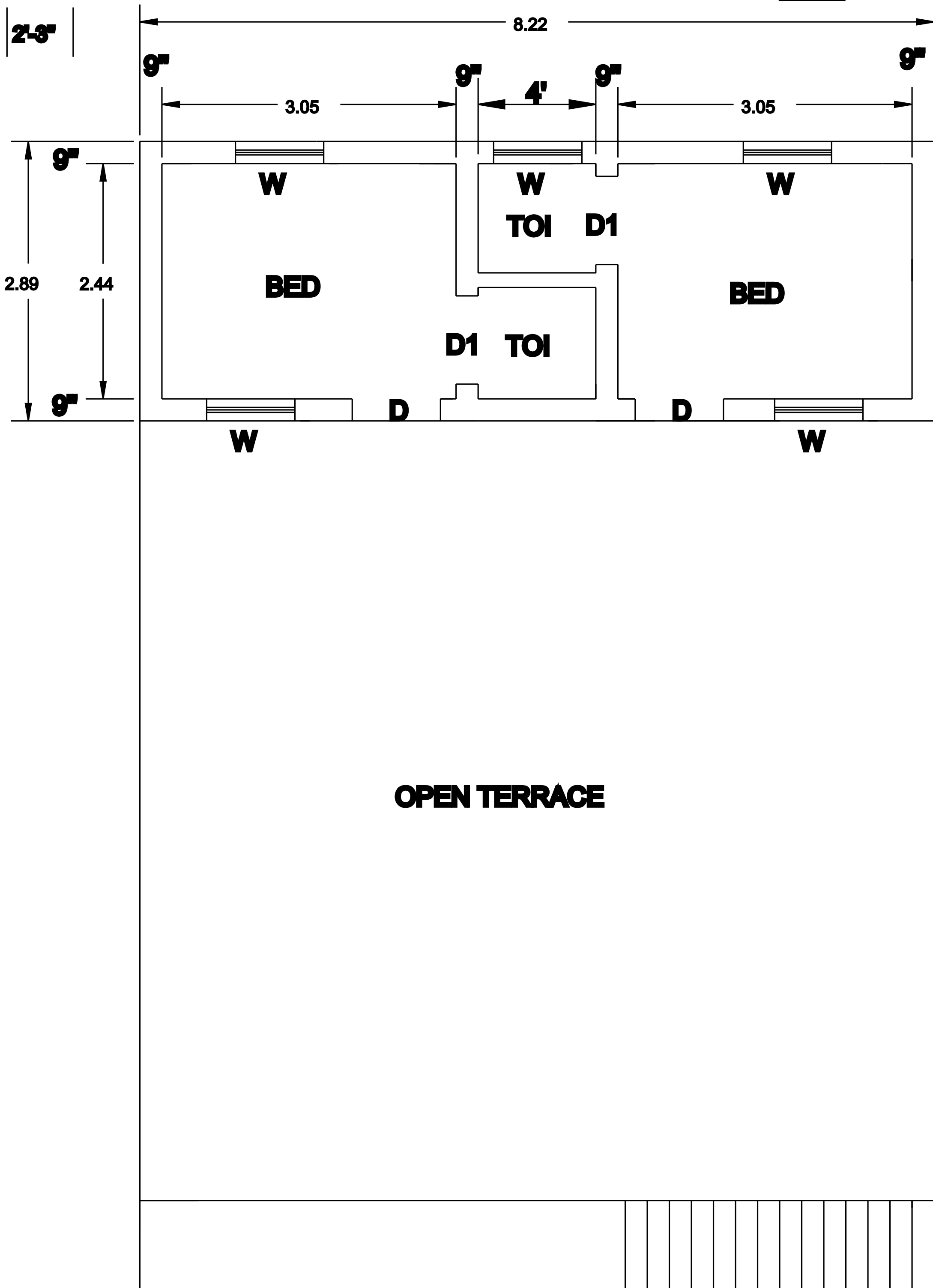
F.F PLAN
