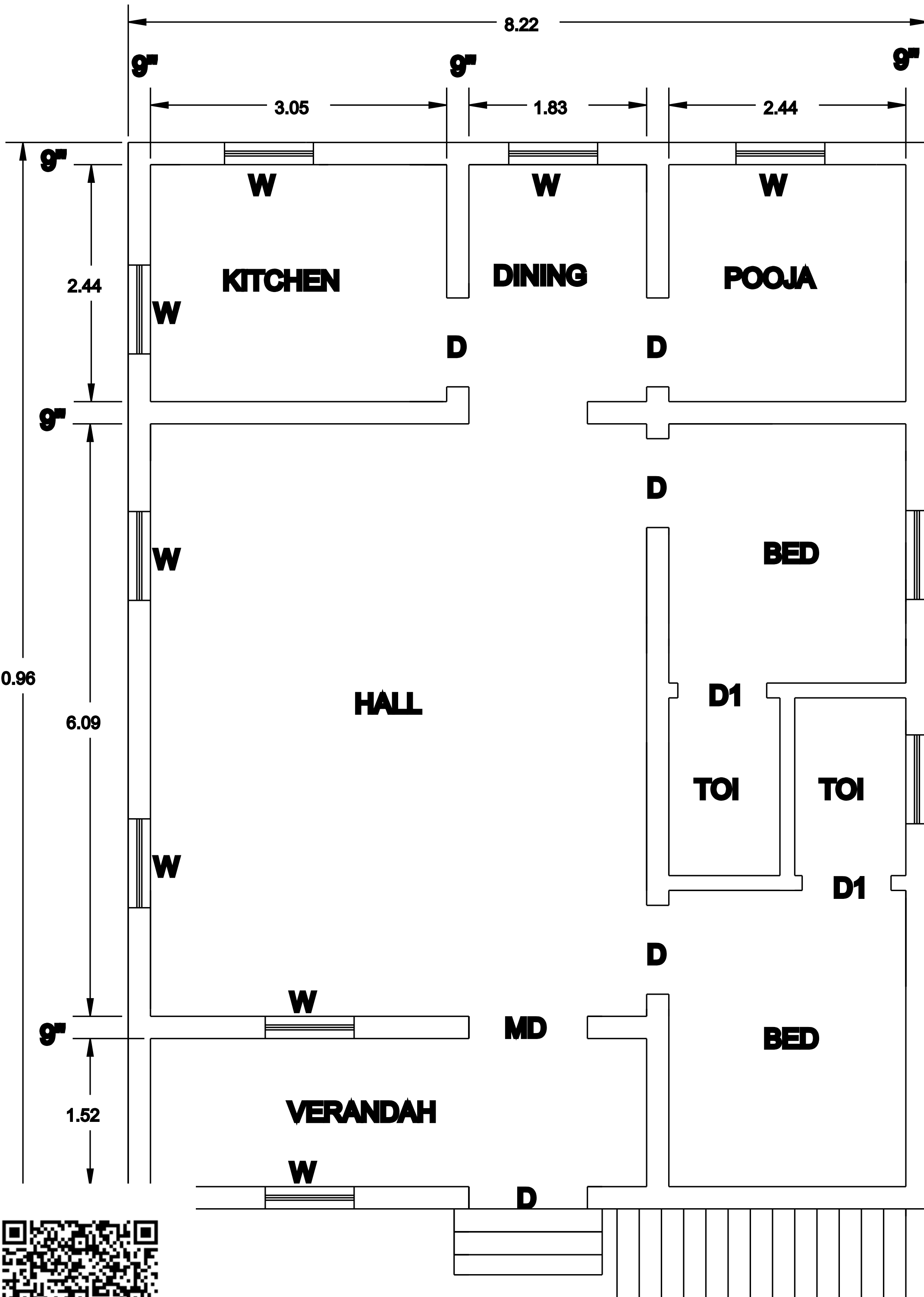
G.F PLAN
