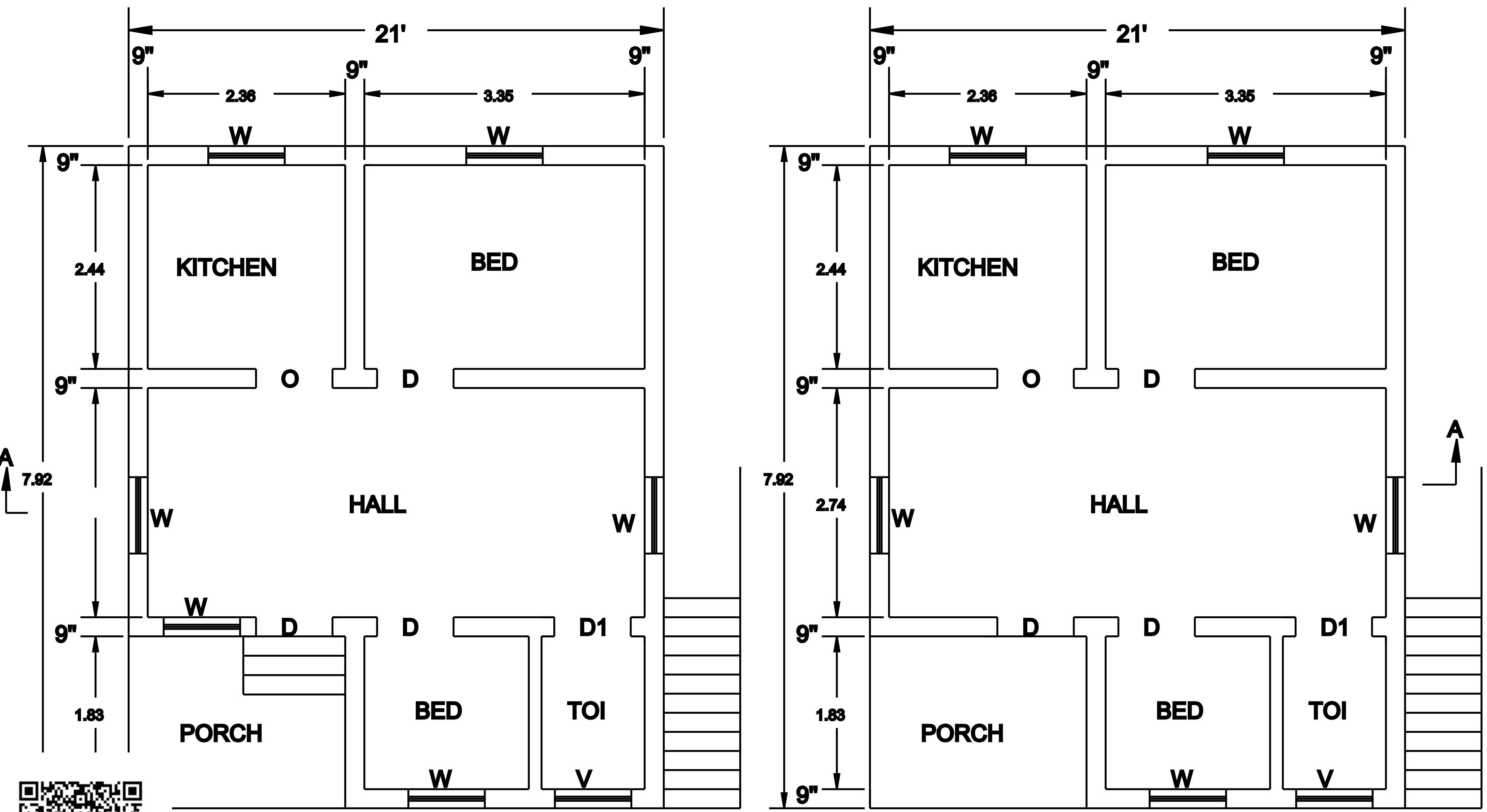
G.F PLAN
