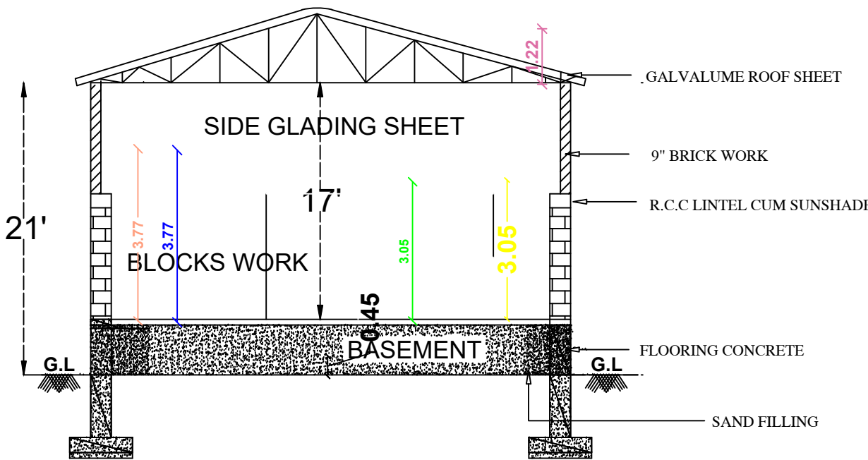
SECTIO ON" AA"
