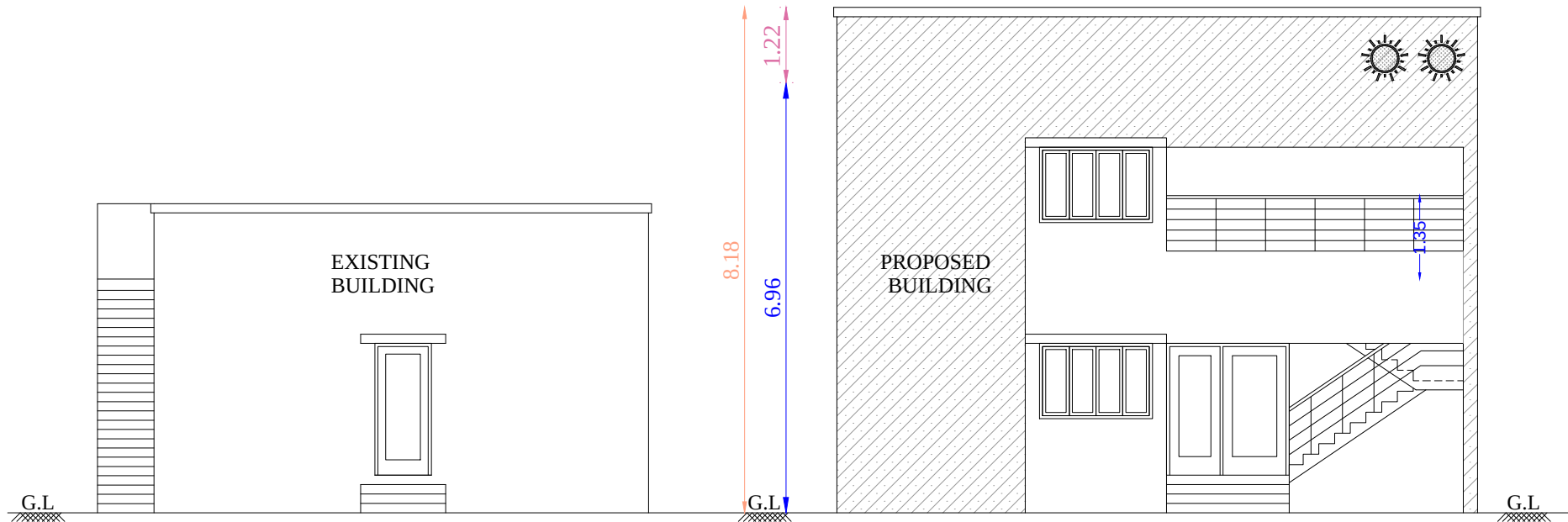
ELEVATION
