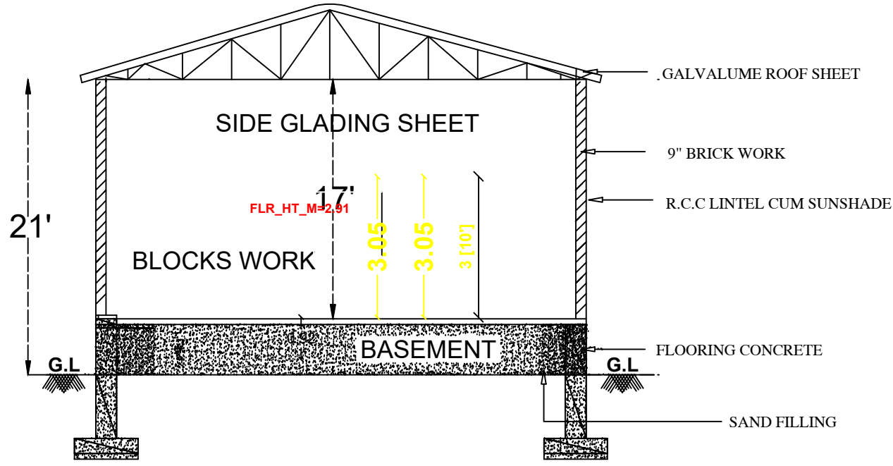
SECTIO ON"AA"
