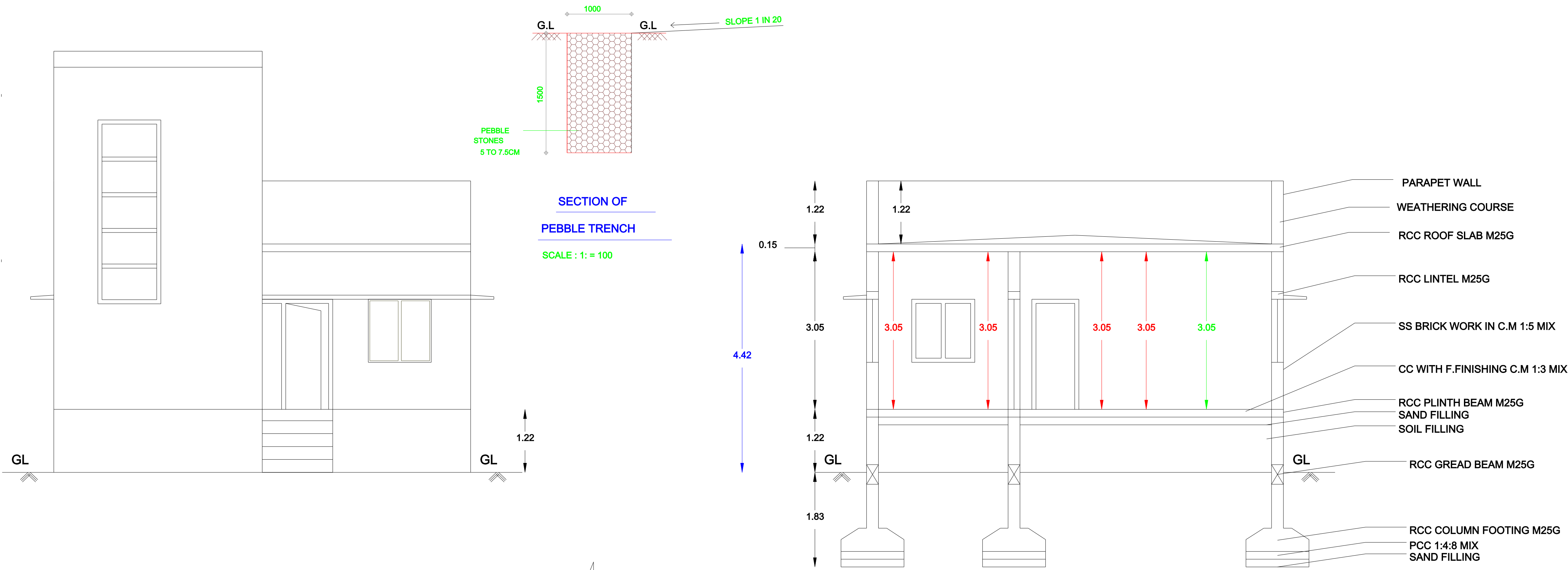
FROND ELEVATION
