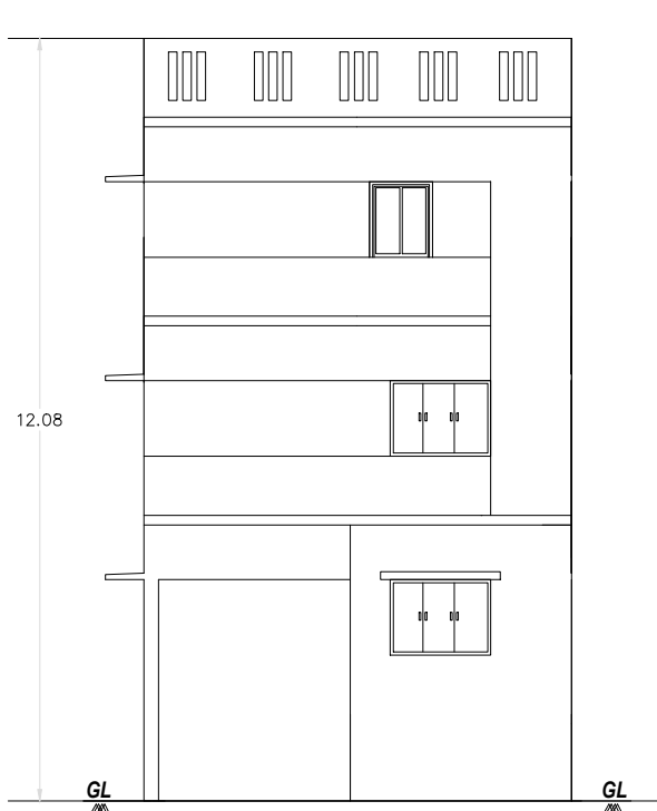
ELEVATION
