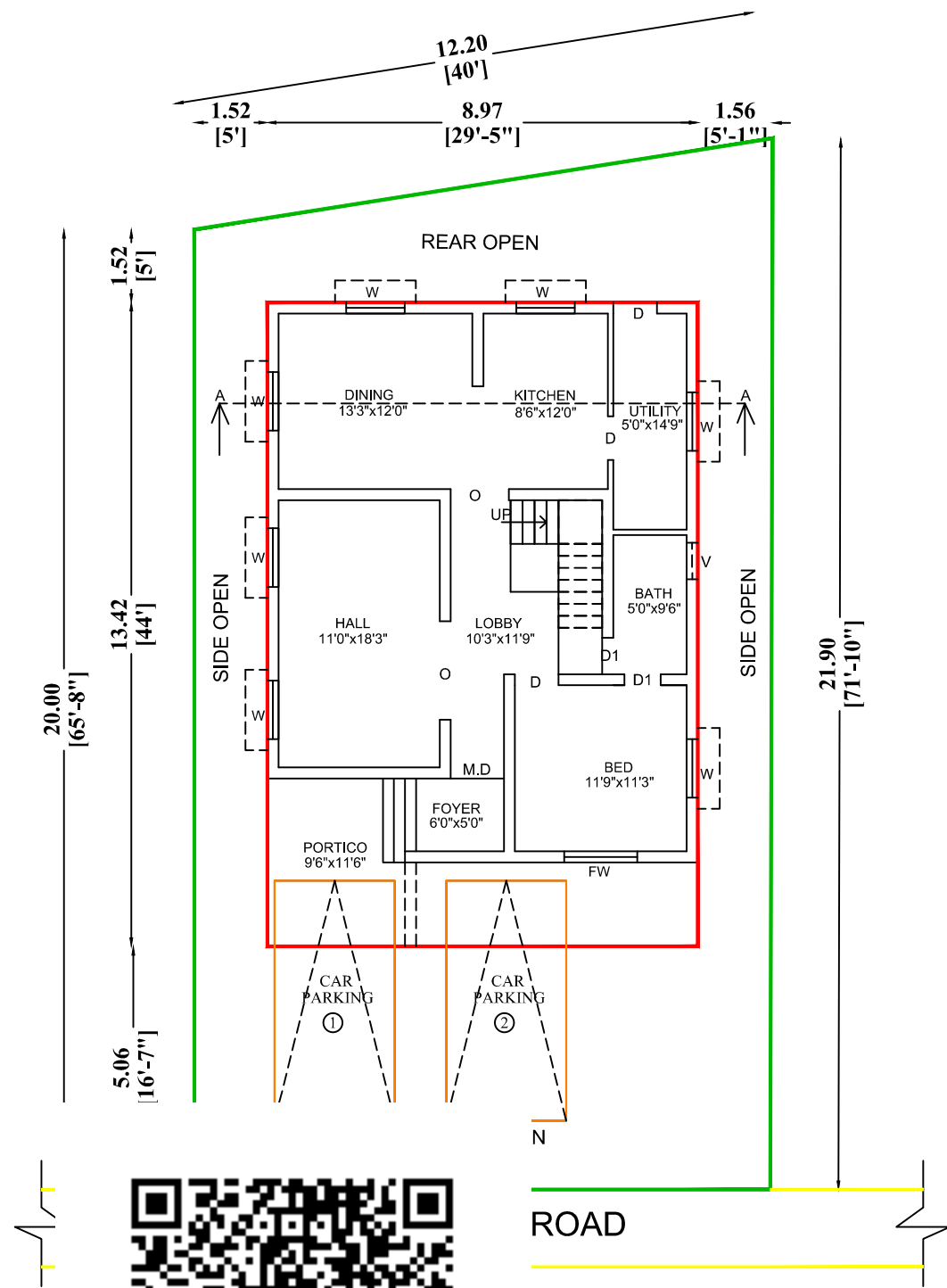
DR PLAN
