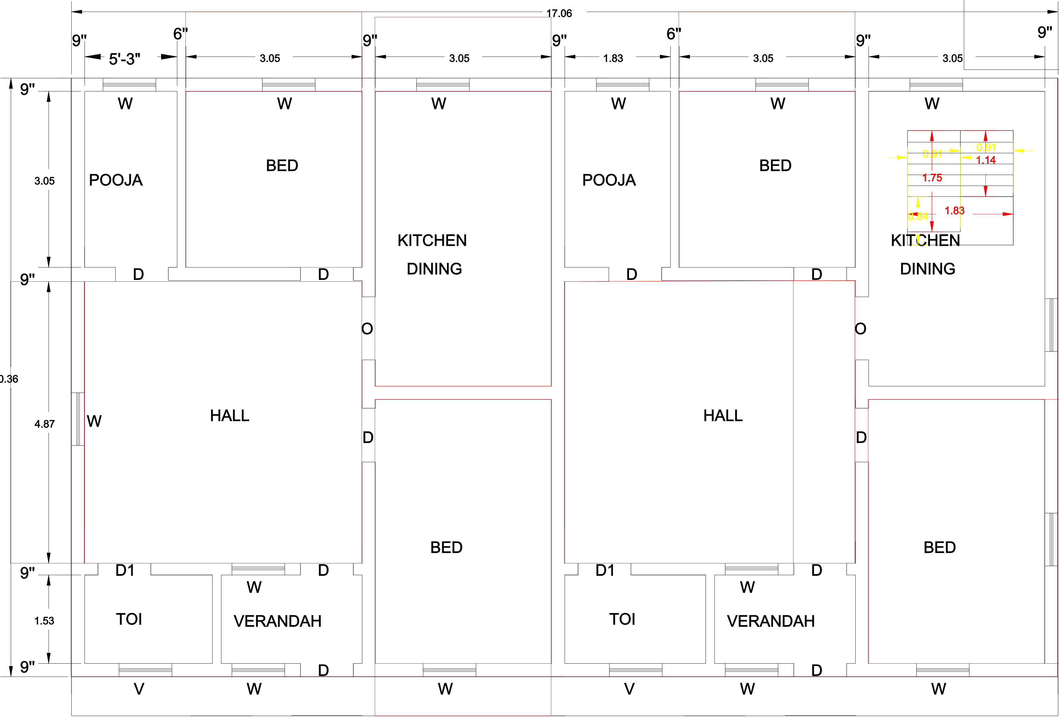
F.F. PLAN
