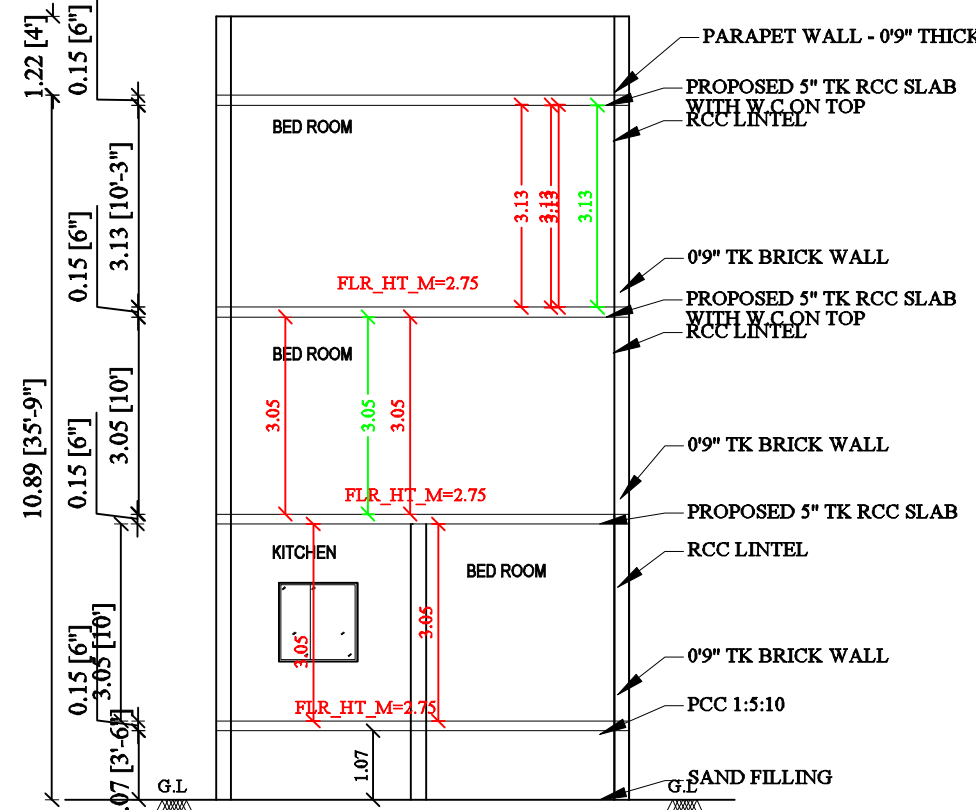
SECTION A-A
