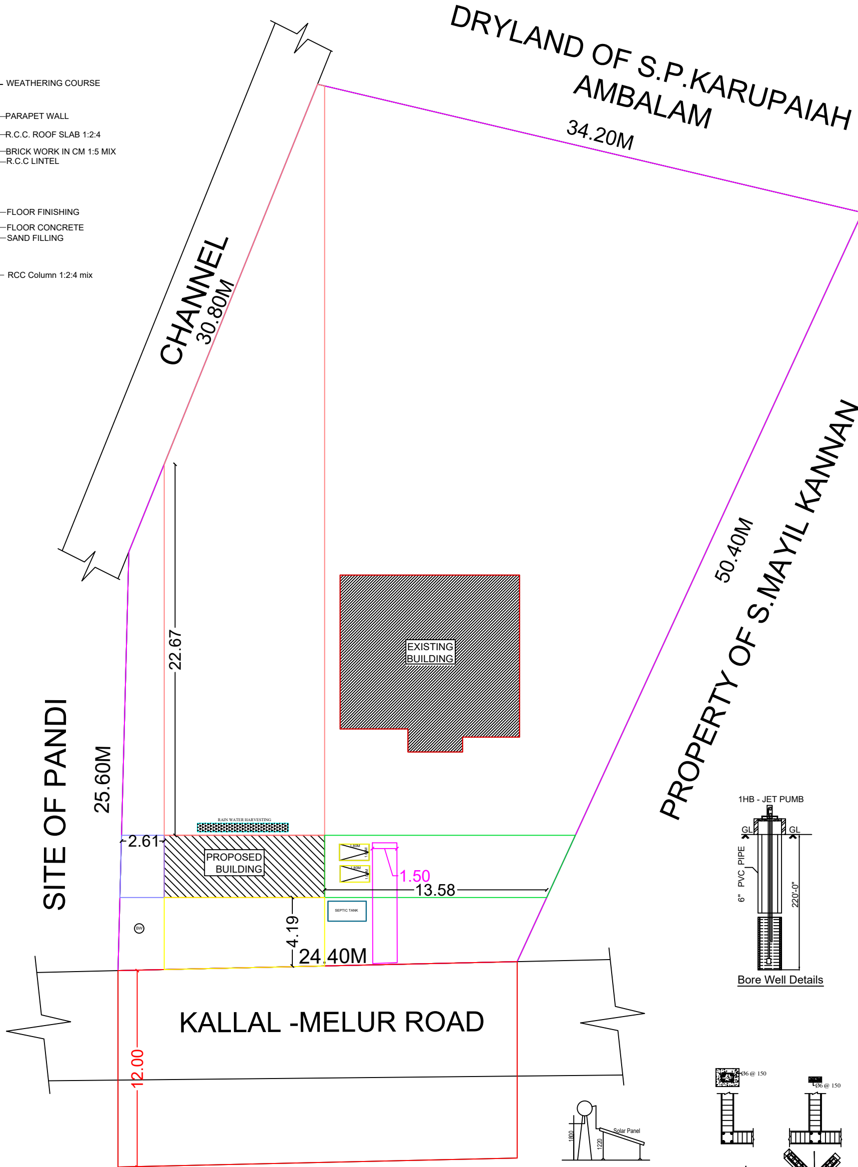
SITE PLAN SCALE : 1:180
