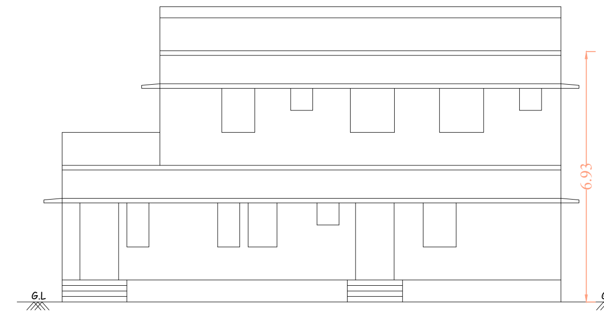
ELEVATION
