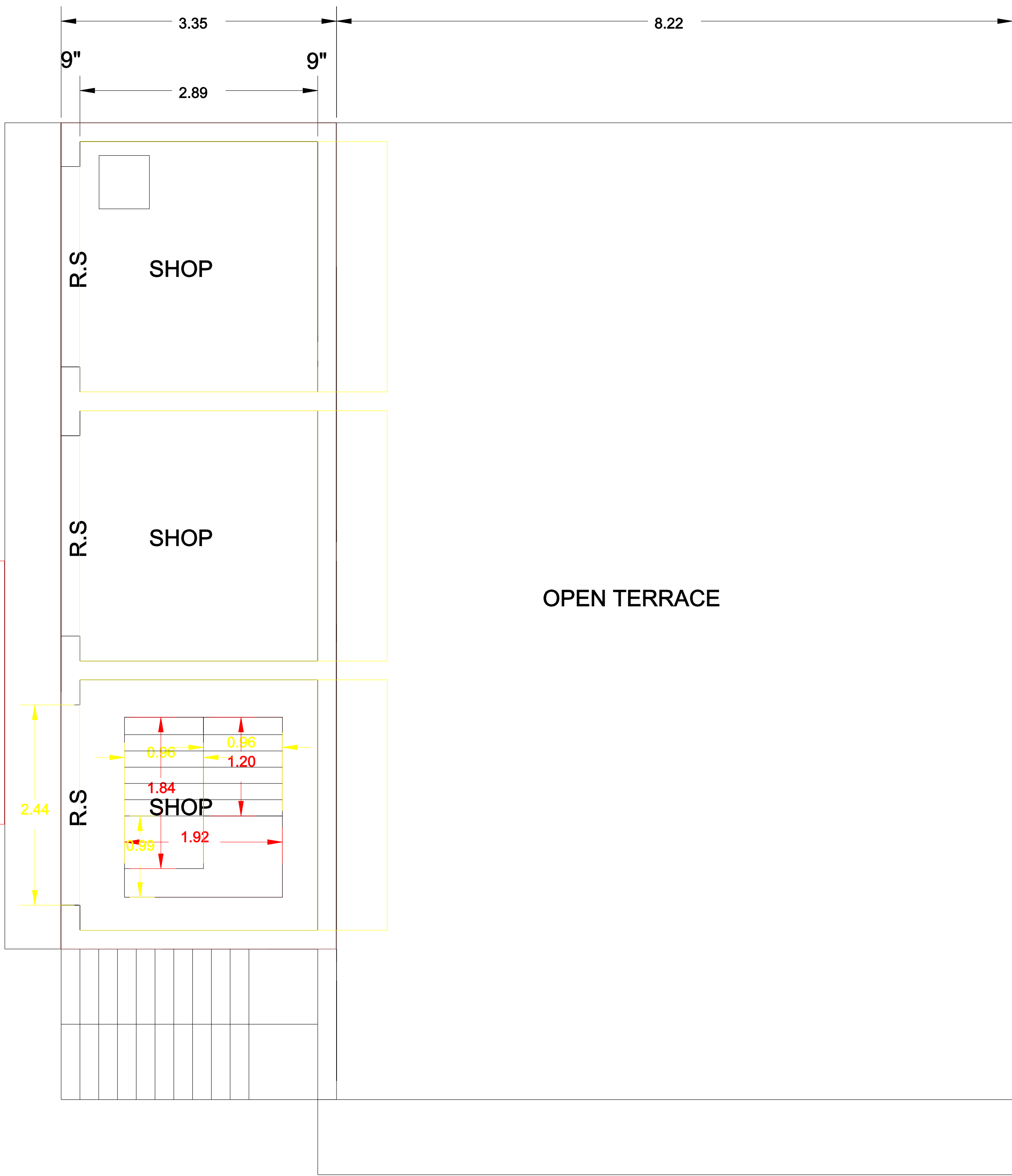
F.F. PLAN
