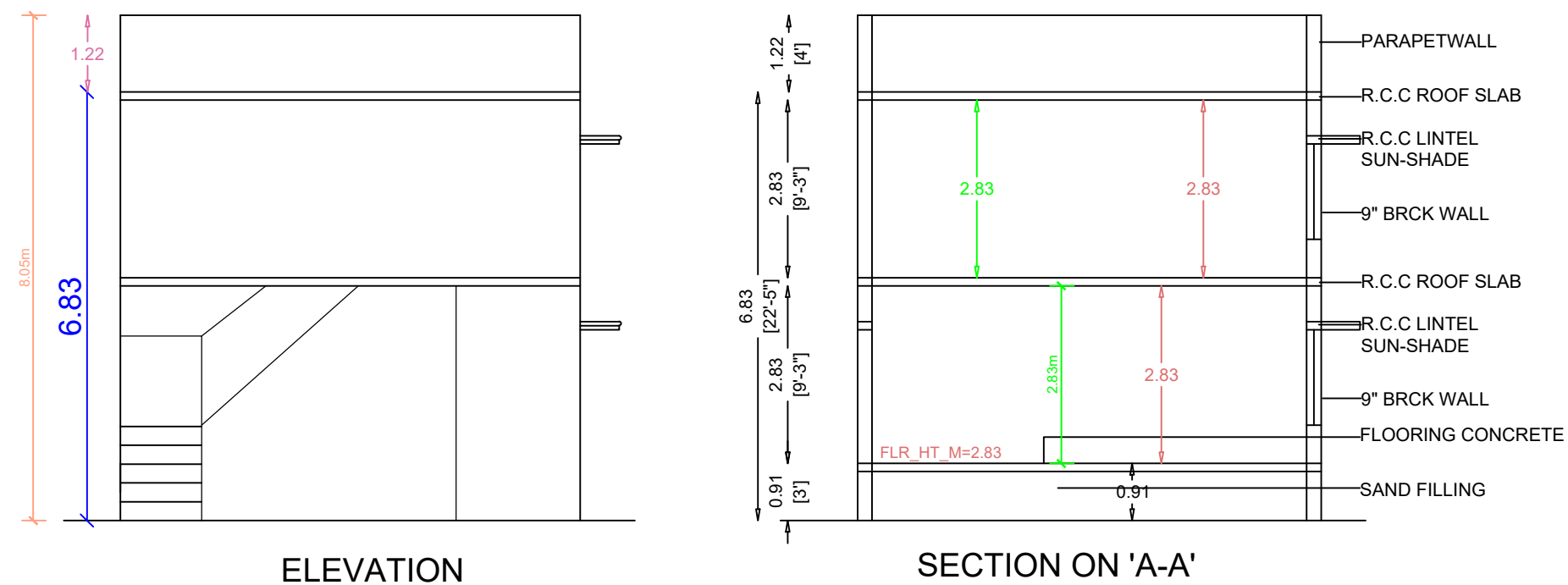
ELEVATION
