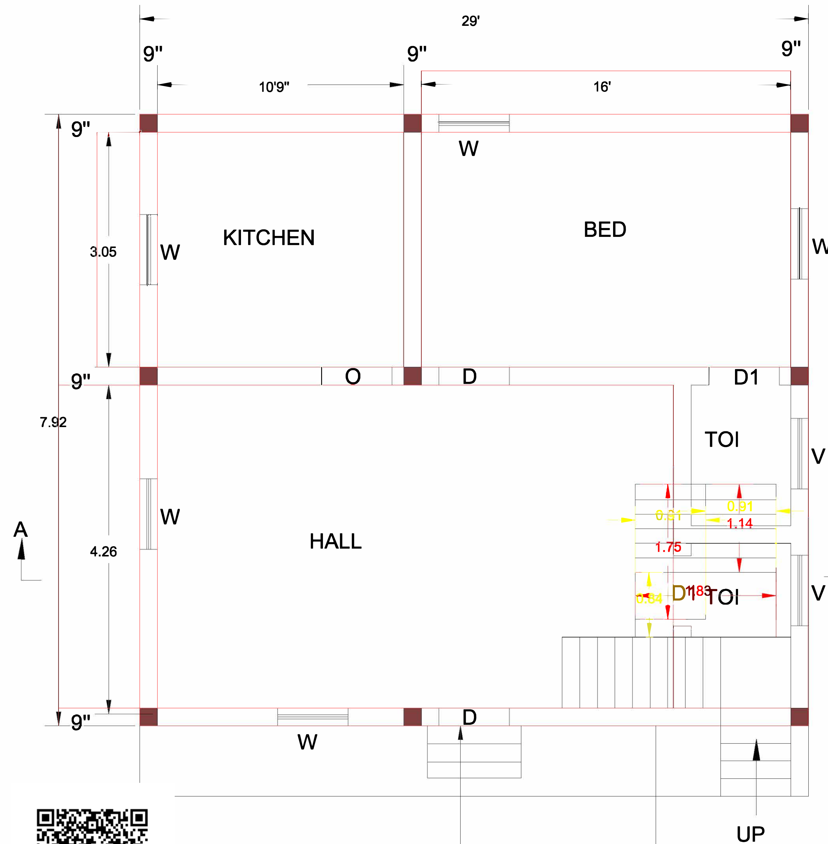
G.F PLAN
