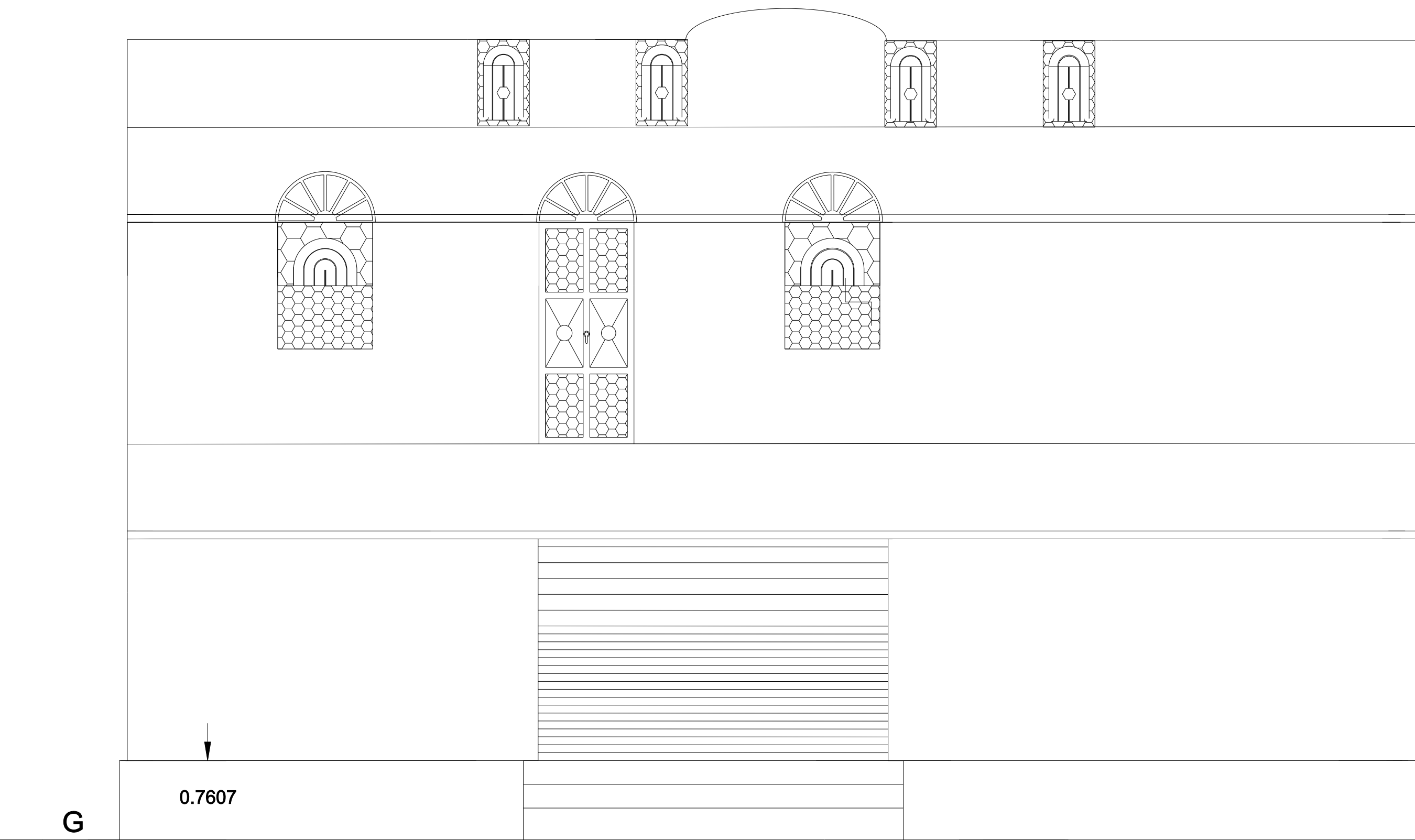
ELEVATION
