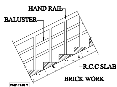
DETAILS OF STAIRCASE (N.T.S)
