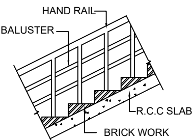
DETAILS OF STAIRCASE (N.T.S)
