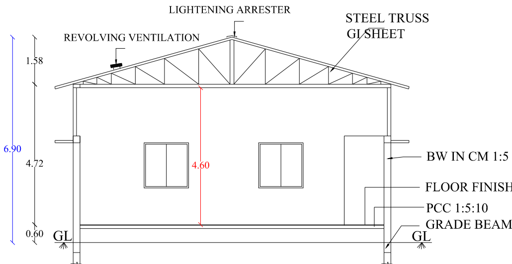
SECTION -XX
