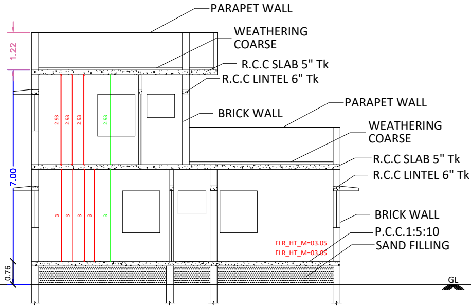
SECTION -AB
