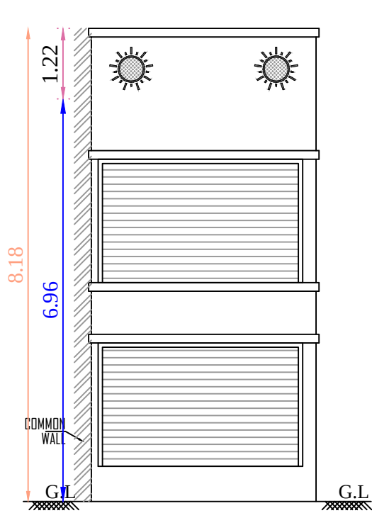
ELEVATION
