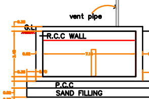
P.C.C SAND FILLING
