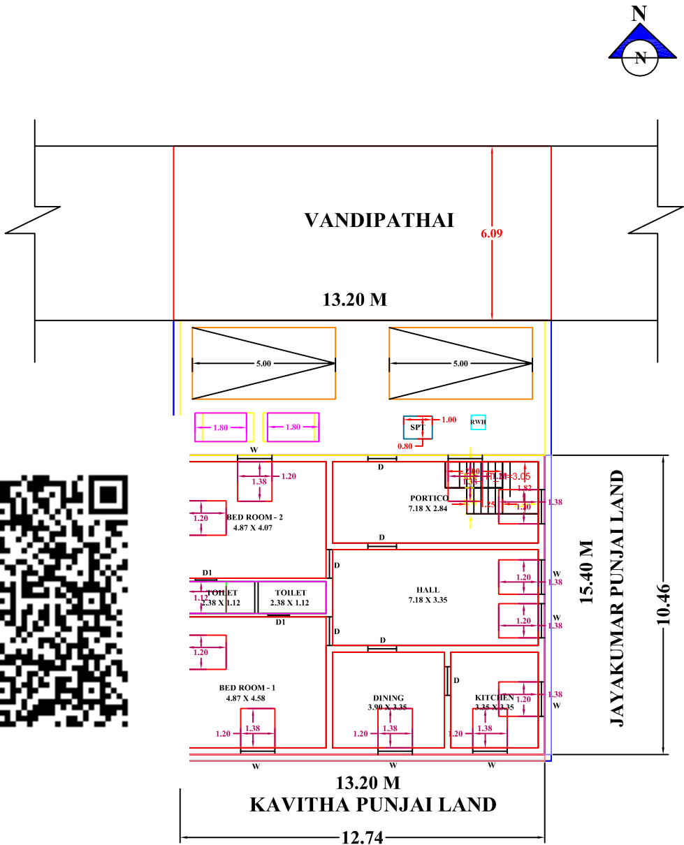
SITE & G.F PLAN
