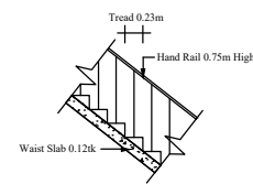
STAIR DETAILS SCALE: 1:50
