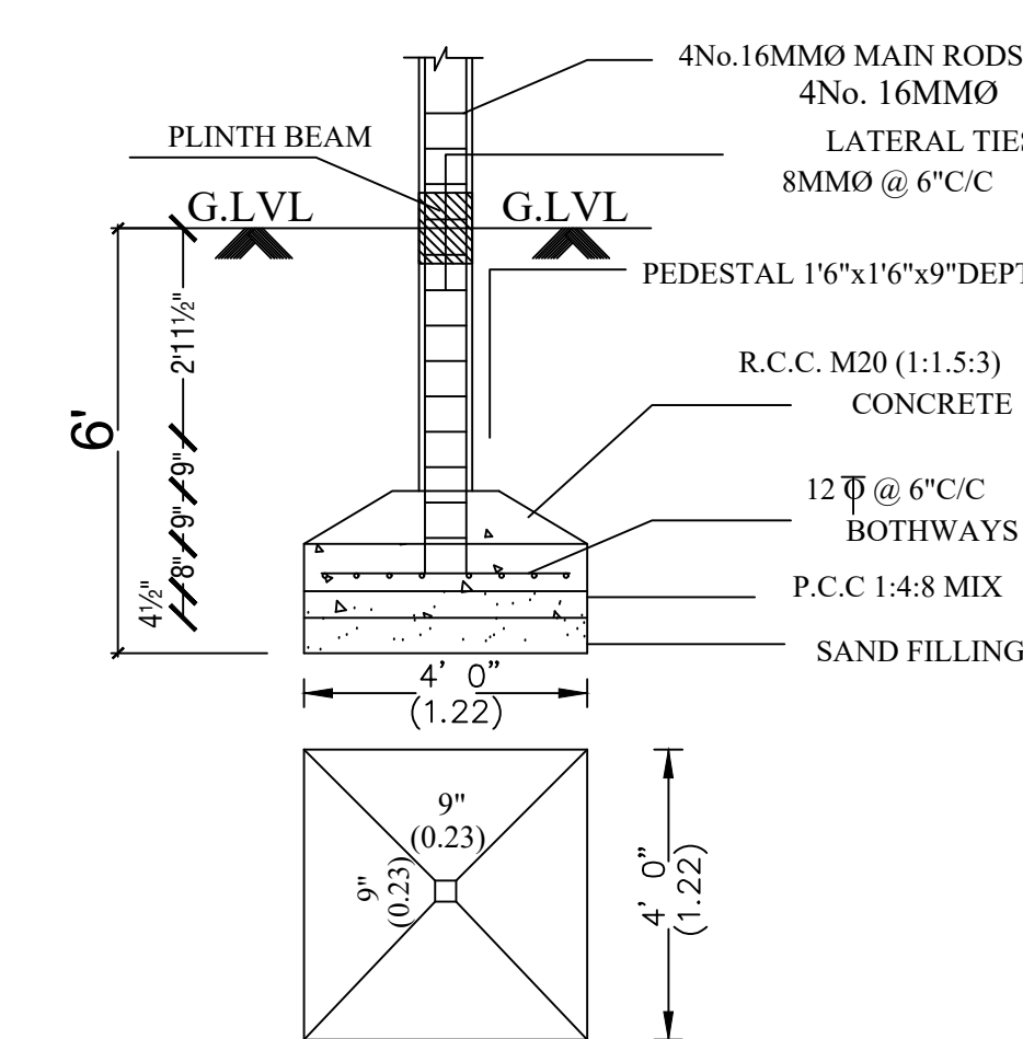
[SCALE: 1:50]
