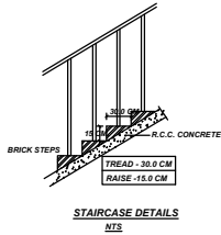
STAIRCASE DETAILS N.T.S
