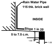
ELEVATION
