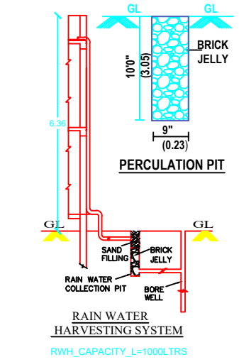
RWH_CAPACITY_L=1000LTRS
