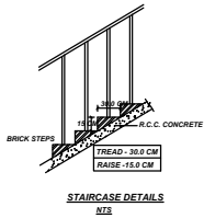
STAIRCASE DETAILS N.T.S.
