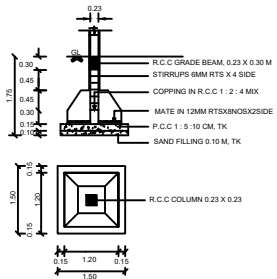
R. C. C. COLUMN DETAILS (1 : 20)
