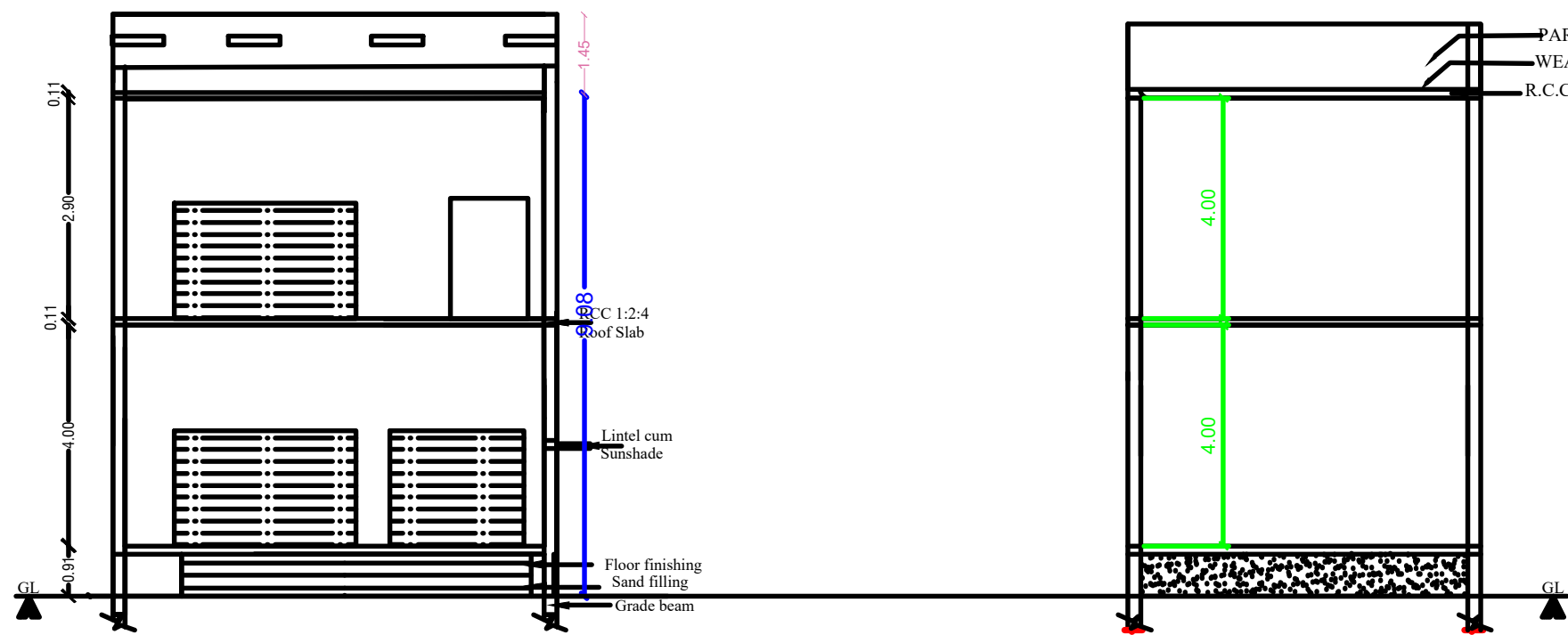
ELEVATION
