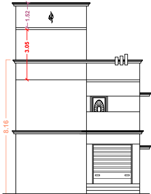
ELEVATION
