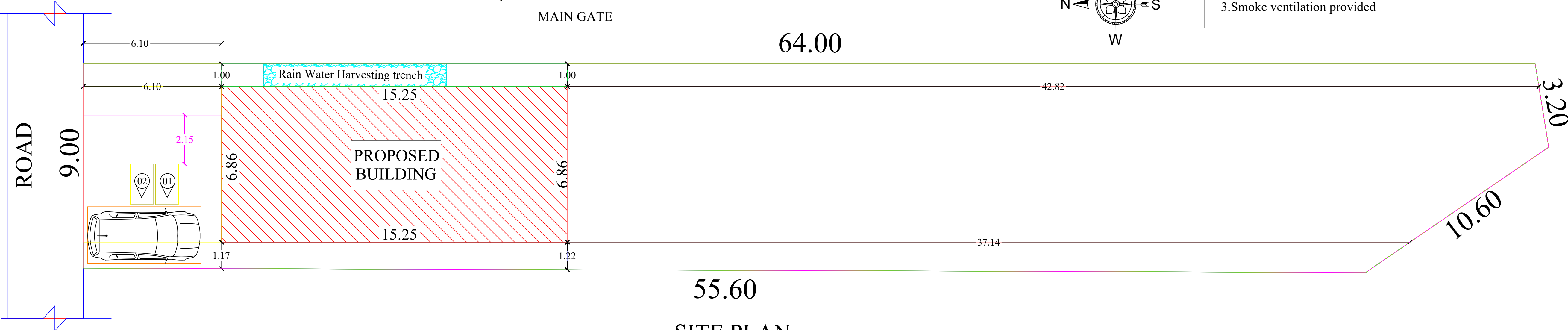
SITE PLAN SCALE 1:100
