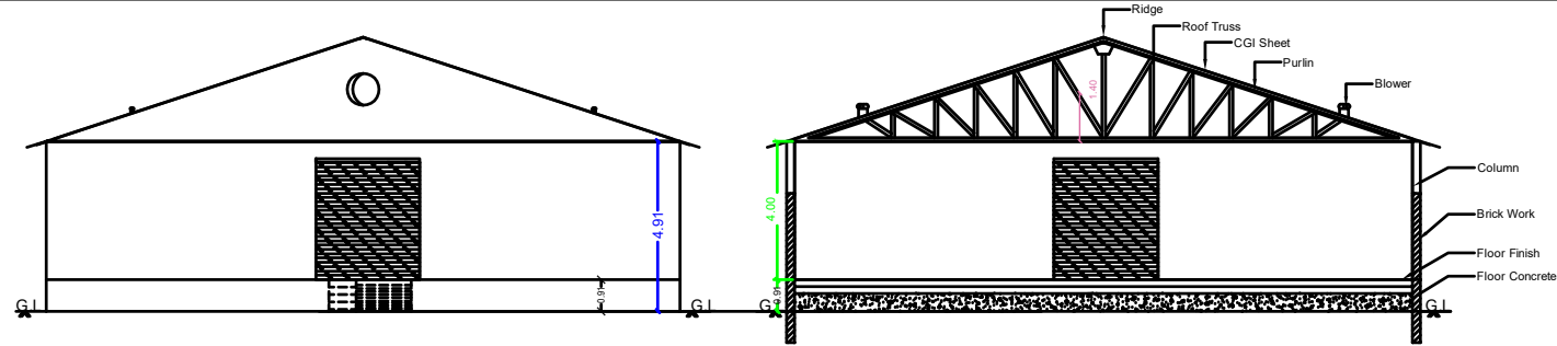
ELEVATION
